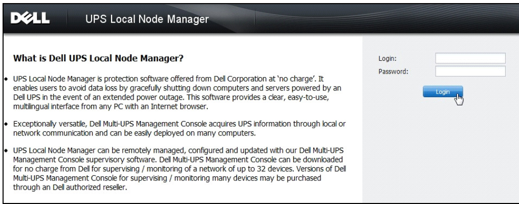
그림 83. 로그인 페이지
